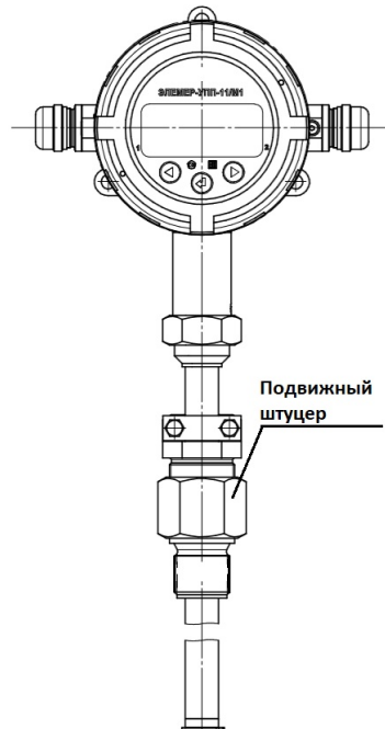
Рисунок В.2 - УПП-11/М1L с подвижным штуцером, индекс за- каза «ПШ»
