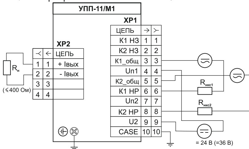
Рисунок Б.3 – Схема электрическая подключений УПП-11/М1, УПП-11/М1L через разъемы ШР с питанием 220 В
