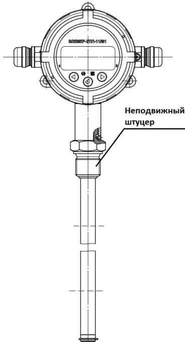
Рисунок В.1 - УПП-11/М1L с неподвижным штуцером, индекс за- каза «-»
