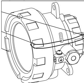
Рисунок А.3 - Место пломбирования УПП-11/М1, УПП-11/М1L
