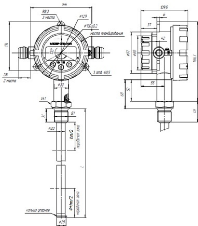
Рисунок А.1 - УПП-11/М1, УПП-11/М1L с неподвижным штуцером
