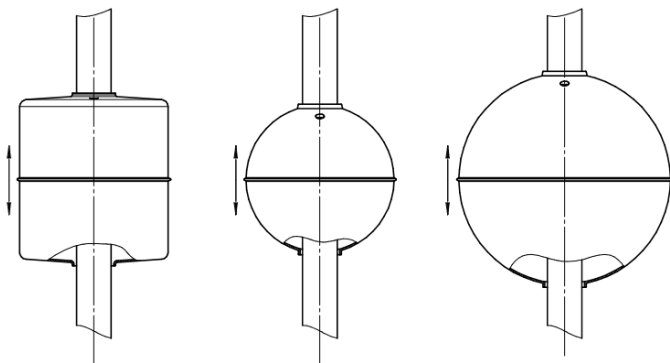
Рисунок 2.3 – Типы поплавков
